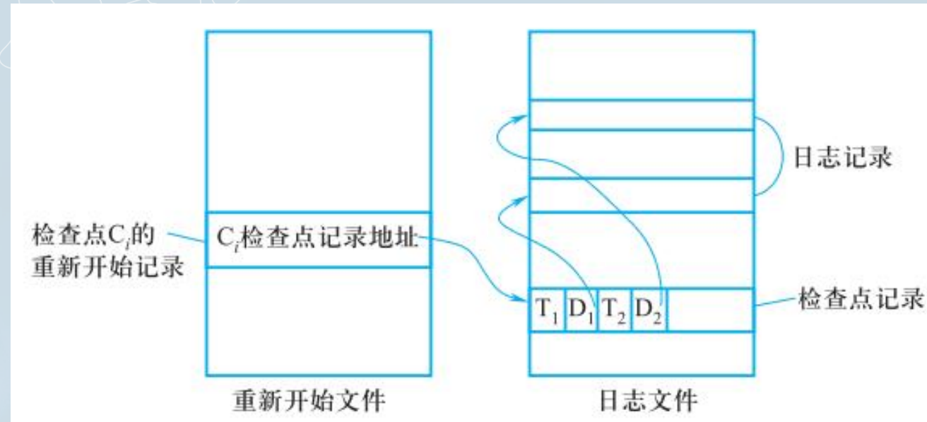
图11.3 具有检查点的日志文件和重新开始文件
